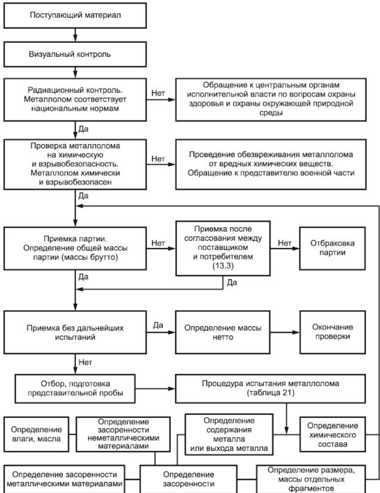
Рисунок 1 - Схема проверки поступающего металлолома
